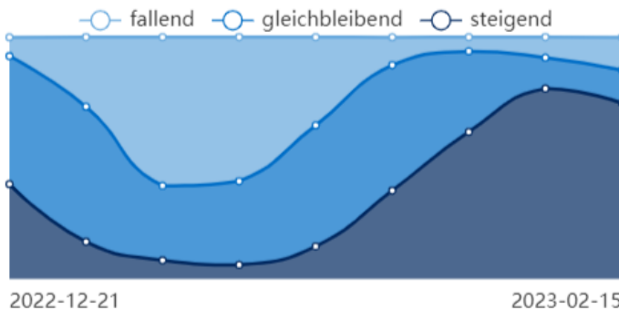
Abbildung 13: Veränderung der SARS-CoV-2-Viruslast im Abwasser, Standorte mit steigendem, gleichbleibendem oder fallendem Trend (Datenstand: 23.02.2023, Quelle: Pandemieradar )
